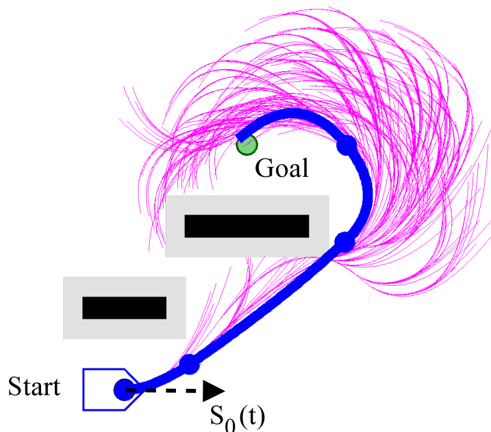
FIGURE 4.24 – Exemple d’un arbre DKP en magenta. La trajectoire sélectionnée par DKP depuis l’état Start jusqu’à l’état Goal apparaît en bleu.
