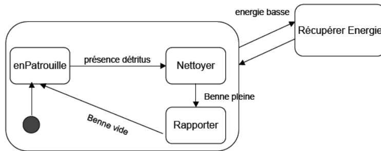
FIG. 1.9 – Exemple d’une machine à états finis hiérarchique reprenant l’exemple de la figure 1.8, tiré du cours “Programmation orientée agents” de Jacques Ferber, Université de Montpellier II.
