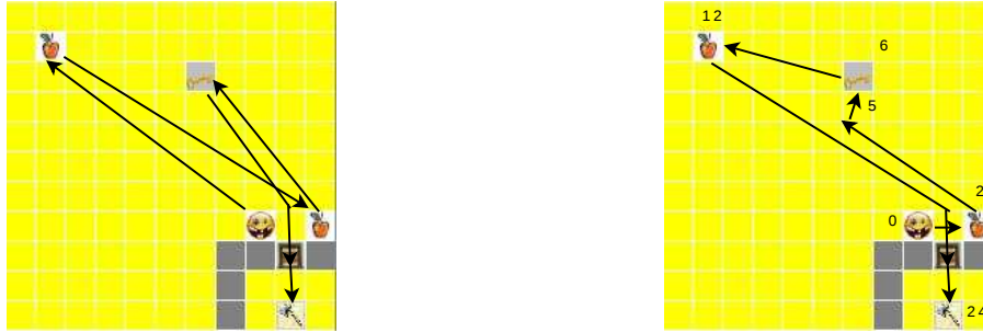
FIG. 5.4 – L'agent a 4 buts, ayant chacun leur propre priorité : prendre pomme1 = 10, prendre pomme2 = 9, prendre clef = 8 et prendre hache = 5. La pomme1 est celle en haut à gauche. La version de droite possède les annotations de pas de temps que l'on retrouve dans la figure 5.5. À gauche, l'ASM prend en compte uniquement la priorité des buts, à droite, il prend en compte la priorité des buts et la motivation de l'opportunisme.
