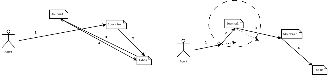
FIG. 3.3 – Schéma de l'étape 1 décrivant l'influence de l'opportunisme. Dans cet exemple, l'agent a reçu deux ordres, l'ordre de prendre et déposer le journal sur la table, l'ordre de prendre et déposer le courrier sur la table, le premier étant plus prioritaire que le second (pour reprendre l'organisation en FIFO des Sims). À gauche , un mécanisme de sélection ne prenant pas en compte l'opportunisme, l'agent exécute les actions dans un ordre très coûteux en déplacement (c'est ce qui se passe dans The Sims). À droite , L'opportunisme influence le comportement de l'agent, étant proche du journal (la notion de proche est représentée par le cercle) l'agent se détourne du courrier pour aller prendre le journal par opportunisme, pour ensuite prendre le courrier (en respectant la priorité des buts). L'agent finit donc par prendre le journal, puis le courrier et les déposer sur la table.
