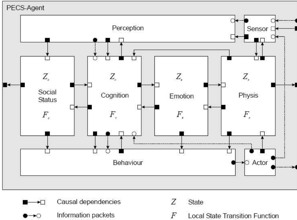
FIG. 1.5 – Architecture d'un agent PECS présentée dans [Sch05].
