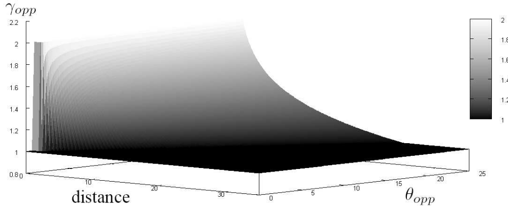
FIG. 3.4 – Les valeurs \gamma_{opp} selon la distance (entre l’agent et la cible) et la valeur de la portée d’influence de l’opportunisme \theta_{opp} . La zone noir représente la neutralité (la cible est trop loin), ce qui signifie que l’opportunisme n’a pas d’influence sur le comportement de l’agent.
