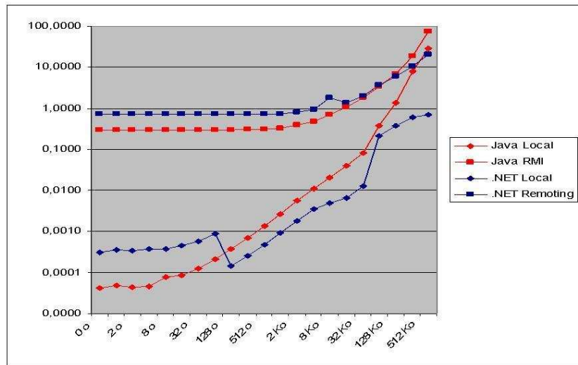
Figure 6.13 – Coût d'un appel de méthode
